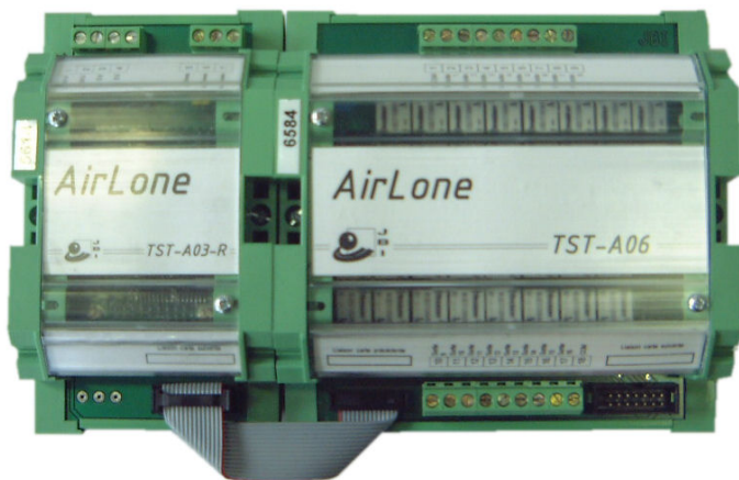
Exemple d'association d'une TST-A03-R avec une TST-A06
